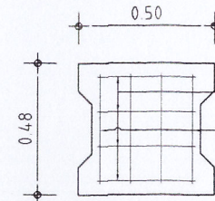
แบบฝาปิดรางระบายน้ำ ค.ล.ล. 1:25
